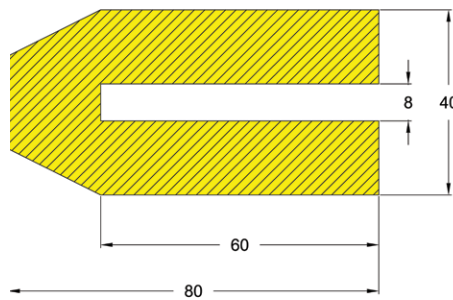
Trapeze 40/80/8
